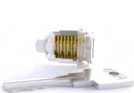
Abb. 1. Sperrstellung
