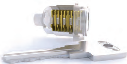
Abb. 1. Sperrstellung
